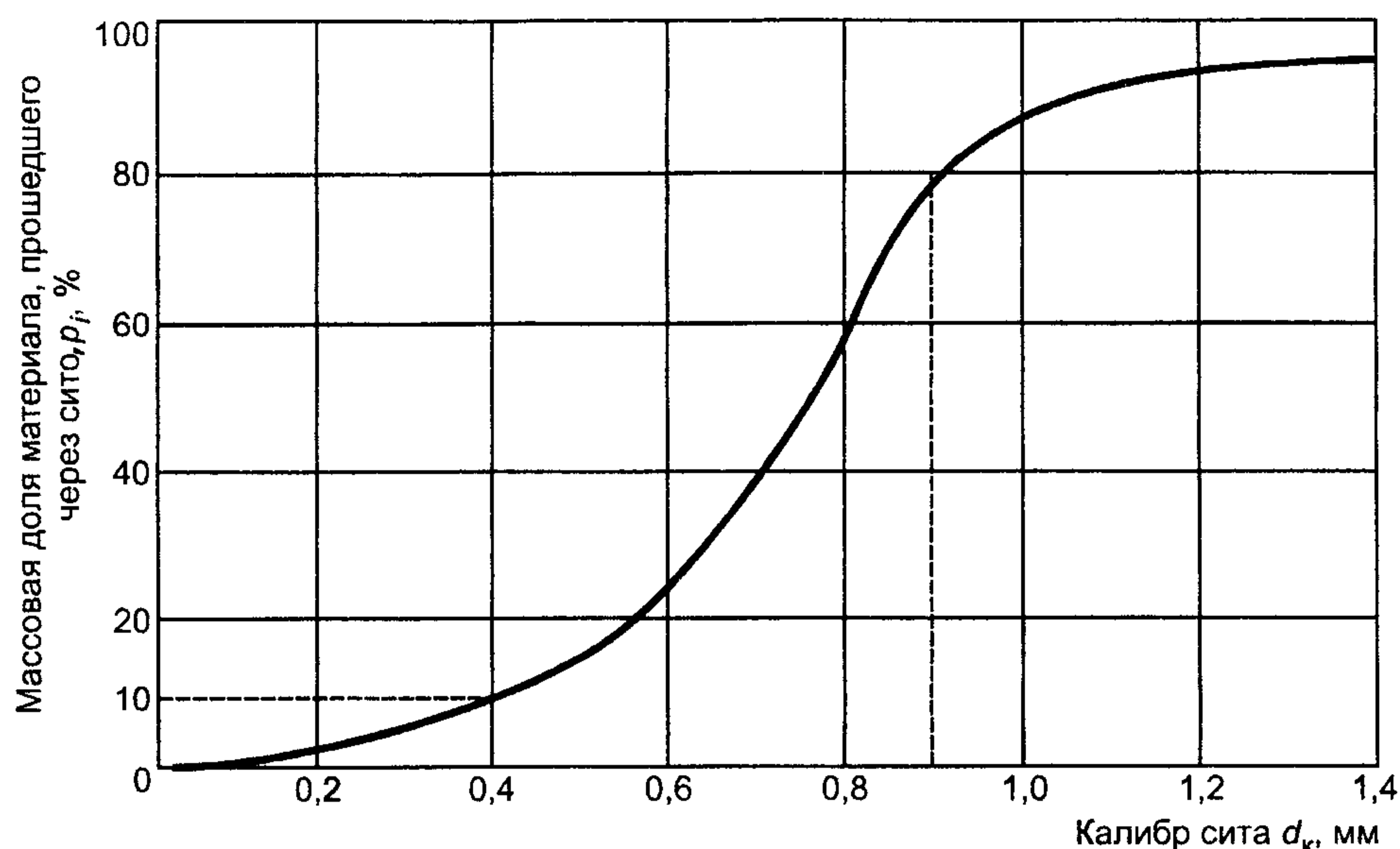
Рисунок А.1 — График ситового анализа материала
